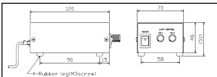
型式:IDV-10D-V / IDV-10D-H(半固定Vr)
