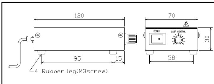
型式:IDV-10S-V / IDV-10S(半固定Vr)
