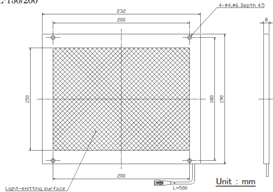
< 生産終了品 > IFL-150/200
